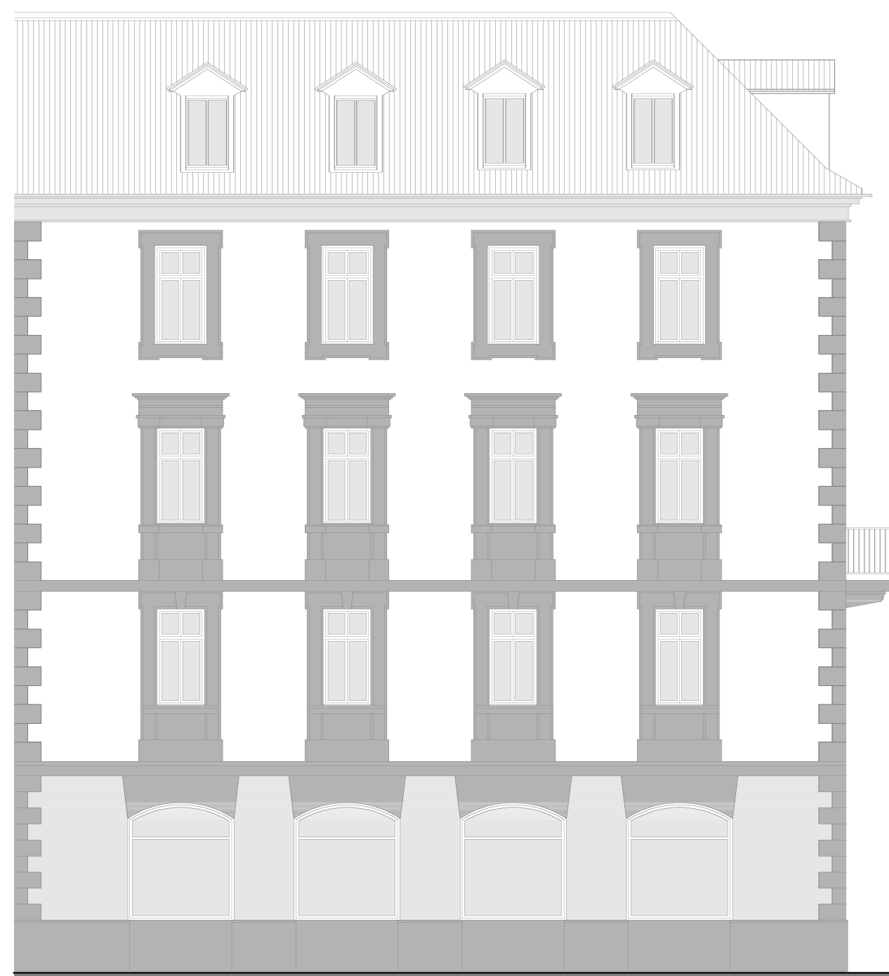
NORDWESTFASADE MAINAUSTRASSE Mst. 1:100
